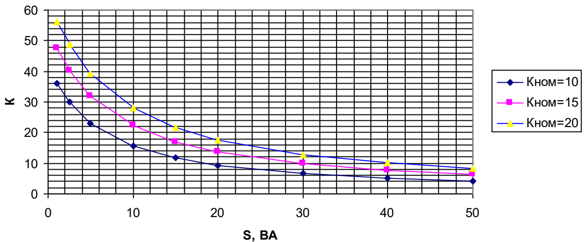
Кривые предельной кратности вторичных обмоток для защиты с классами точности 5Р и 10Р и номинальной нагрузкой 15 ВА трансформаторов с первичным током 1500А
