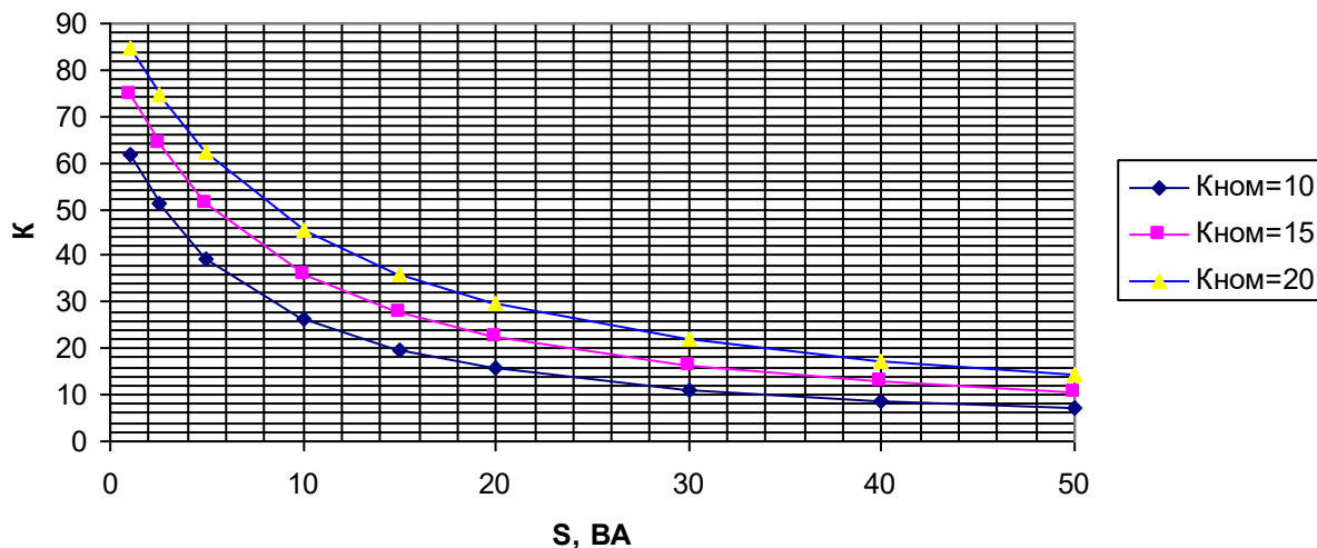
Кривые предельной кратности вторичных обмоток для защиты с классами точности 5Р и 10Р и номинальной нагрузкой 30 ВА трансформаторов с первичным током 1000А
