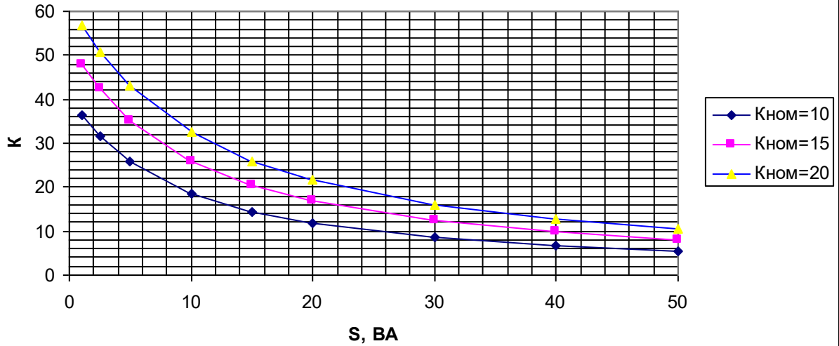
Кривые предельной кратности вторичных обмоток для защиты с классами точности 5P и 10P и номинальной нагрузкой 20 ВА трансформаторов с первичным током 2000А
