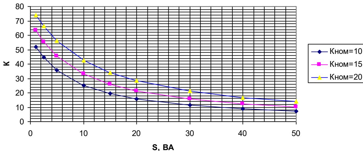
Кривые предельной кратности вторичных обмоток для защиты с классами точности 5Р и 10Р и номинальной нагрузкой 30 ВА трансформаторов с первичным током 1500А
