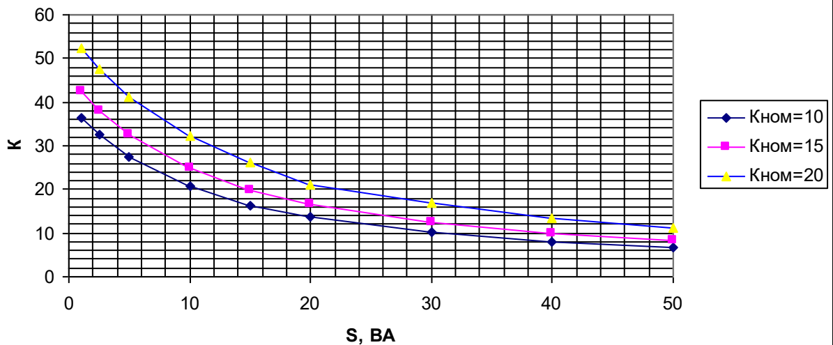
Кривые предельной кратности вторичных обмоток для защиты с классами точности 5P и 10P и номинальной нагрузкой 20 ВА трансформаторов с первичным током 2500А
