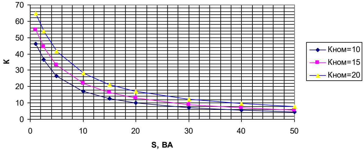
Кривые предельной кратности вторичных обмоток для защиты с классами точности 5Р и 10Р и номинальной нагрузкой 15 ВА трансформаторов с первичным током 1000А
