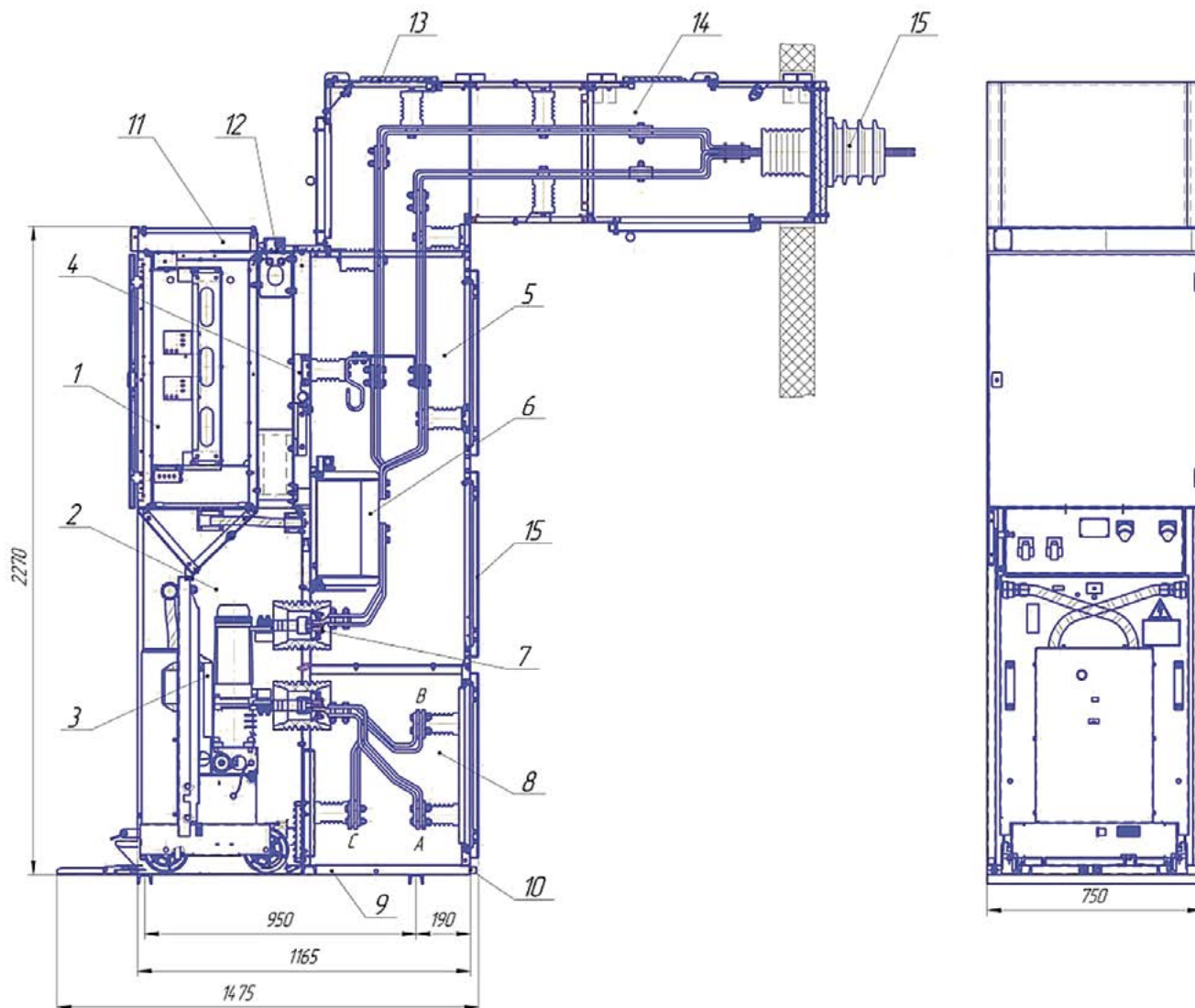
Рисунок 1 Шкаф шинного ввода (вывода)
